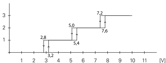
Diagram: Výkonové stupně ventilátoru pro přívodní napětí 0-10V, 3 stupně
