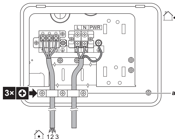
a Kabelová příchytká
