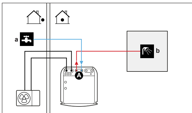
A Teplá užitková voda a VSTUP studené vody
