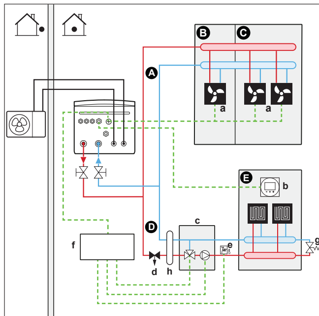
3 Systém s hydraulickým separátorem pro obě zóny: Pro tento systém je vyžadováno přímé čerpadlo pro doplňkovou zónu.
