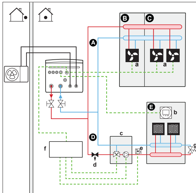
2 Systém s hydraulickým separátorem pro hlavní zónu:
