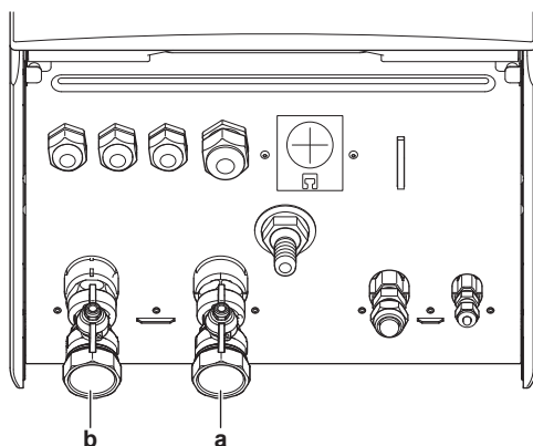
a Přívod vody b Odvod vody
